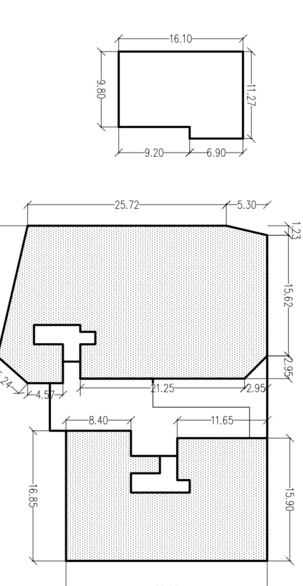
PIANTA A QUOTA +0,00
