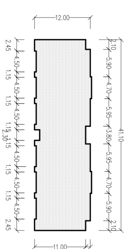
PIANTA A QUOTA +3,50, 6,50, 9,50, 12,50
