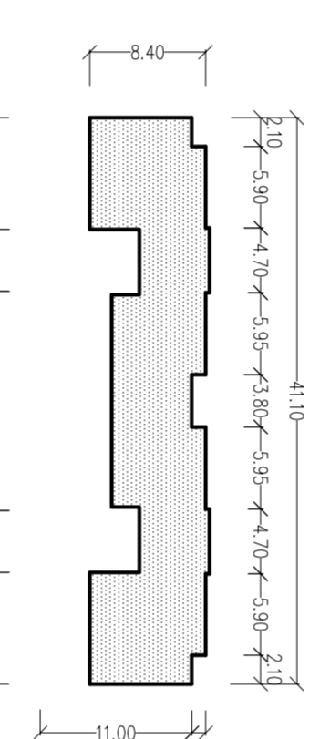
PIANTA A QUOTA +0,10
