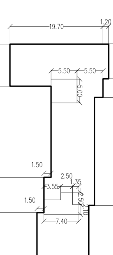
PIANTA A QUOTA +0,20
