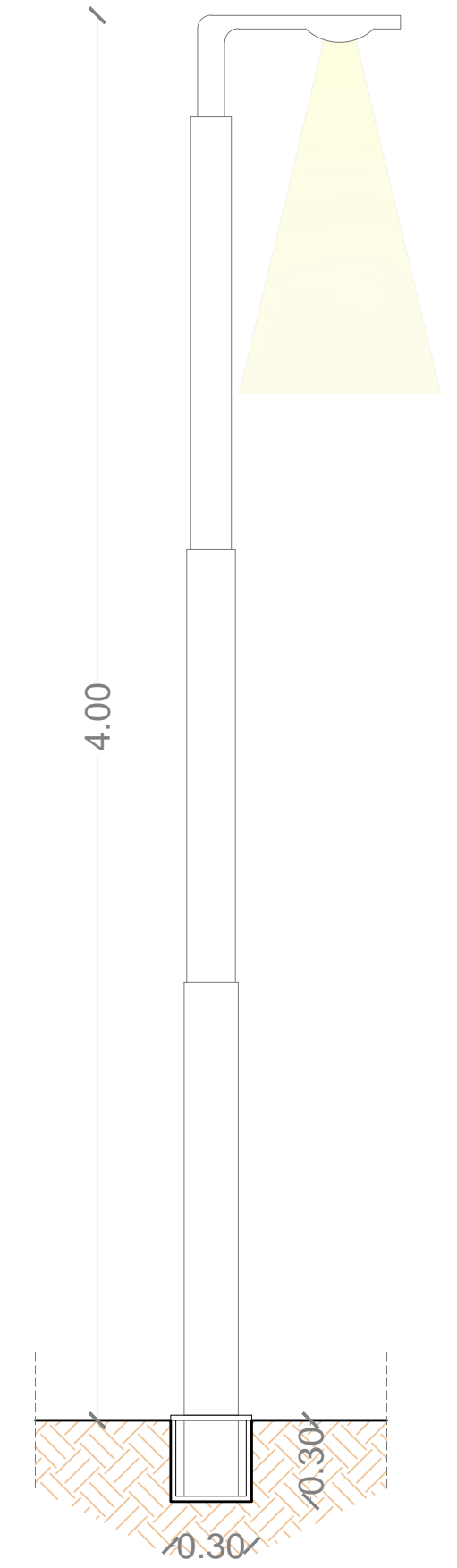
DETTAGLIO palo per illuminazione pubblica scala 1:50
